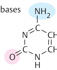
Cytosine (Cyt)
