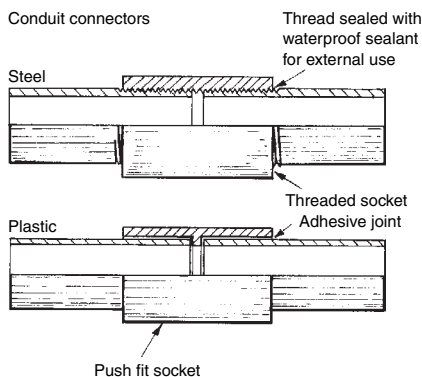
Conduit connectors
