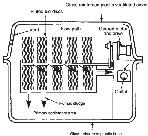
Longitudinal section
